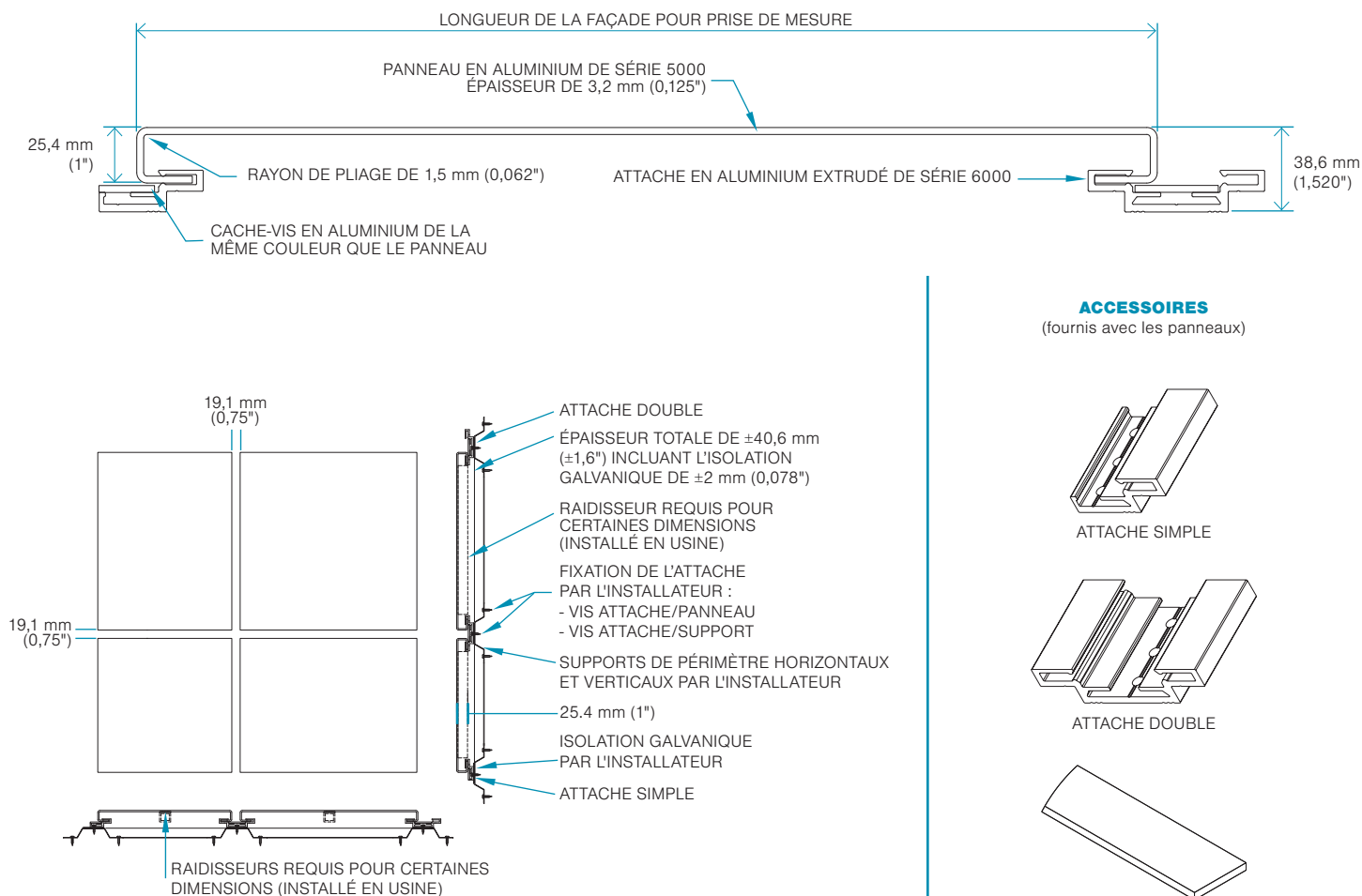
CACHE-VIS DE 25,4 mm (1") ET DE 31,75 mm (1,25")
